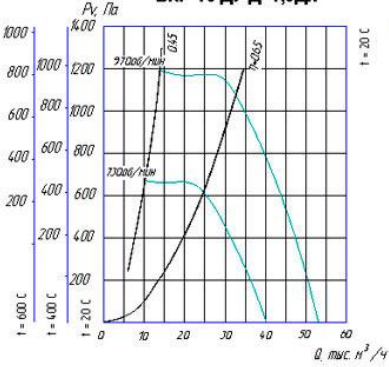
ВКР-12,5 ДУ Д=1,0Дн
