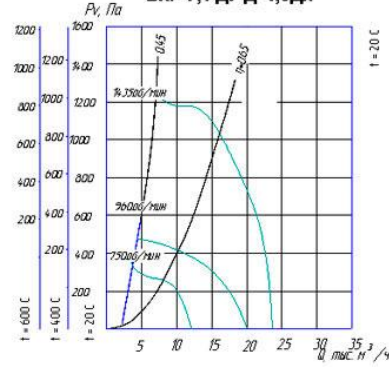
ВКР-9 ДУ Д=1,0Дн
