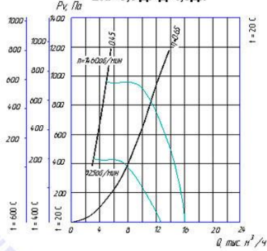
ВКР-8 ДУ Д=1,0Дн
