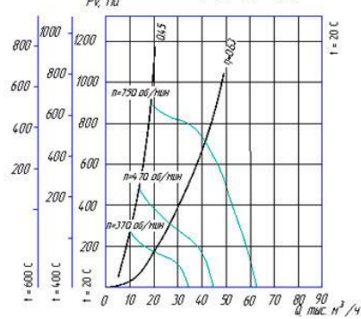
ВКР-12,5 ДУ Д=1,0Дн
