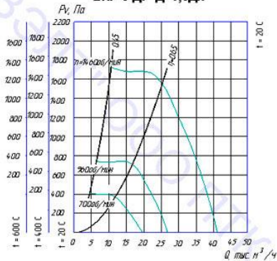
ВКР-10 ДУ Д=1,0Дн
