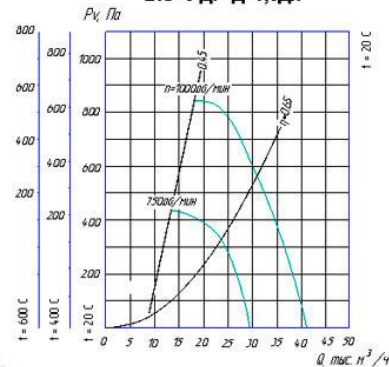
ВКР-11,2 ДУ Д=1,0Дн
